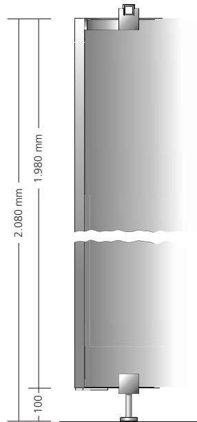
1 Höhengschnitt Front
