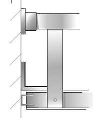
5 Wandanschluss
