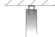
5 Wandanschluss mit U-Profil als Schattenfuge
